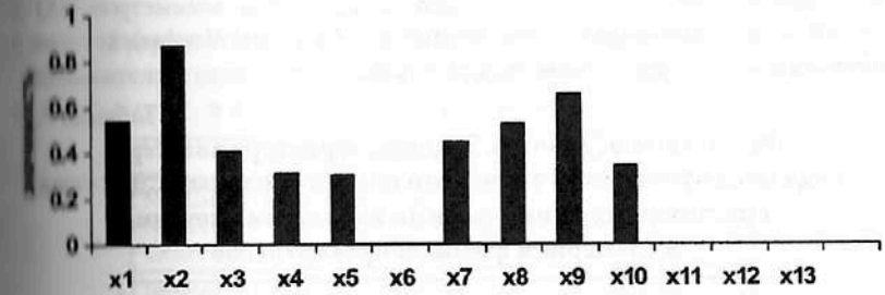
компоненты x_i параметров углеводно-липидного обмена, определяющие вектор состояния организма человека
