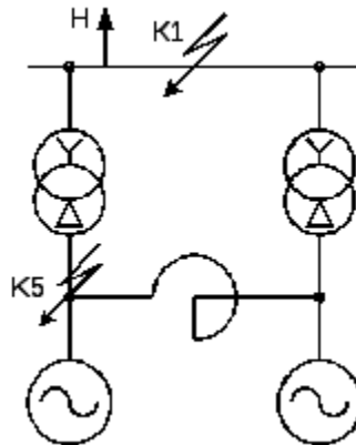
Рис. 4.2. Схема станции № 1
