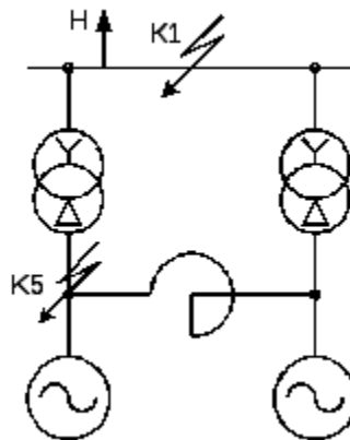
Рис. 1 Схема станции № 1
